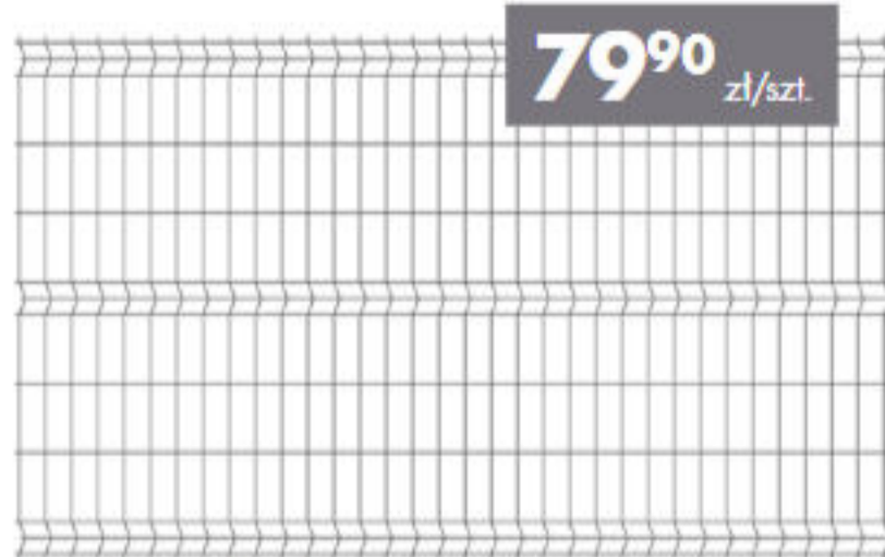
Panel ogrodzeniowy wys. 1,52 m, wym. oczka 50x200 mm, śr. drutu 4 mm, ocynk + RAL 7016 połysk
